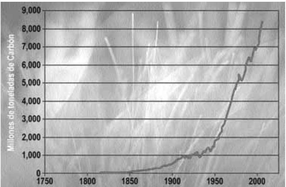
Emisión mundial de dióxido de carbón por combustión de energías por fósiles 1751-2006
